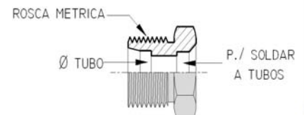
ROSCA MACHO - MÉTRICA ASIENTO VIROLA
