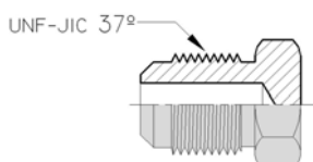
ROSCA UNF JIC 37°
