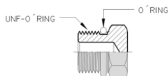
ROSCA UNF ASIENTO O RING
