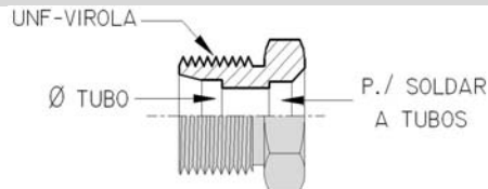
ROSCA UNF ASIENTO VIROLA
