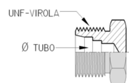
MACHO ROSCA UNF ASIENTO VIROLA
