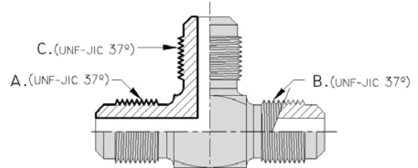
CON UNF ASIENTO JIC 37° EN TODOS LOS EXTREMOS
