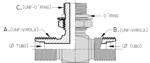
UNF VIROLA - UNF O´RING (centro) UNF VIROLA
