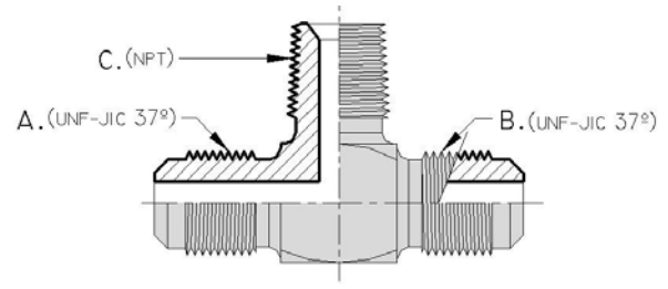
UNF JIC 37° - UNF JIC 37° ROSCA NPT CÓNICA (CENTRO)
