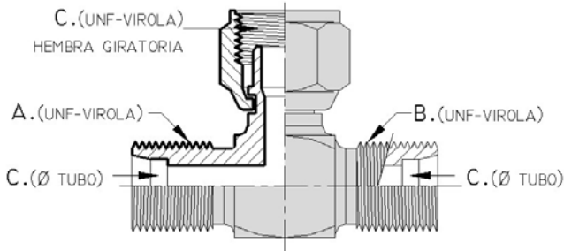
CON ALOJAMIENTO VIROLA EN LOS EXTREMOS A Y B HEMBRA GIRATORIA VIROLA (centro)
