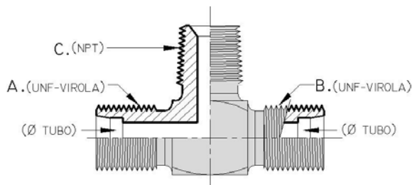
CON ALOJAMIENTOS ASIENTO VIROLA EN A Y B ROSCA NPT CÓNICA (CENTRO)
