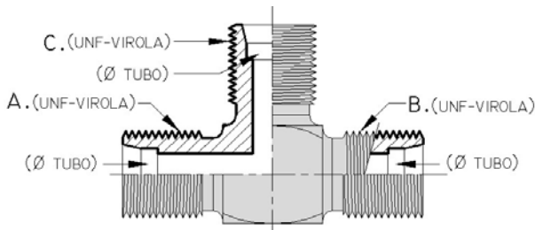
CON ALOJAMIENTO VIROLA EN TODOS LOS EXTREMOS
