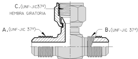
UNF JIC 37° - UNF JIC 37° - H. GIRATORIA UNF JIC 37° (centro)
