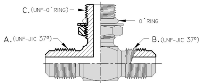
UNF JIC 37° - UNFJIC 37° - UNF MACHO O´RING (centro)
